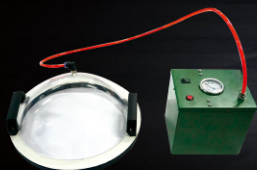
真空测漏仪
